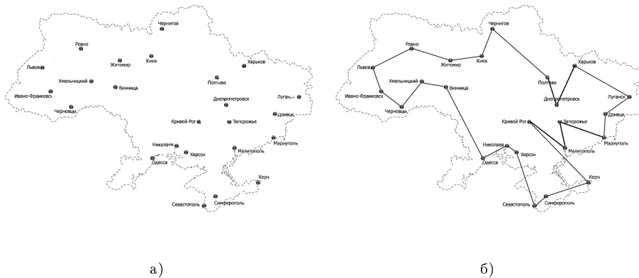
Рис. 4 Иллюстрация результатов применения алгоритма упорядочивания.
